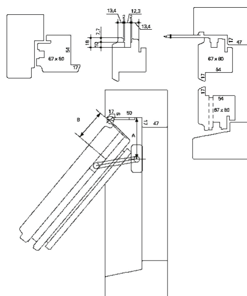
Positie remschaar bij uitzetramen Remschaar op stijl
