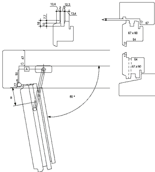
Positie remschaar bij draairamen Remschaar op boven- of onderdorpel
