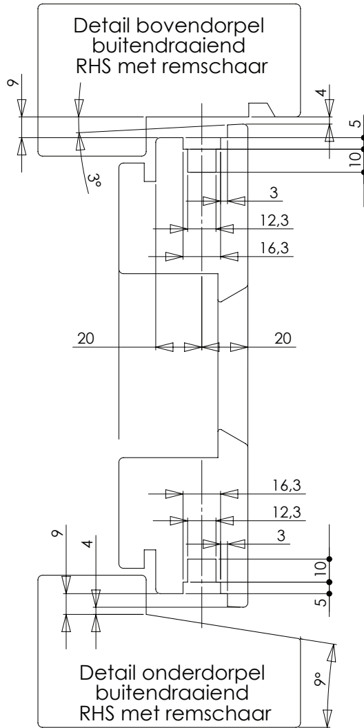
Voorbeeld freestekening Raambeslag
