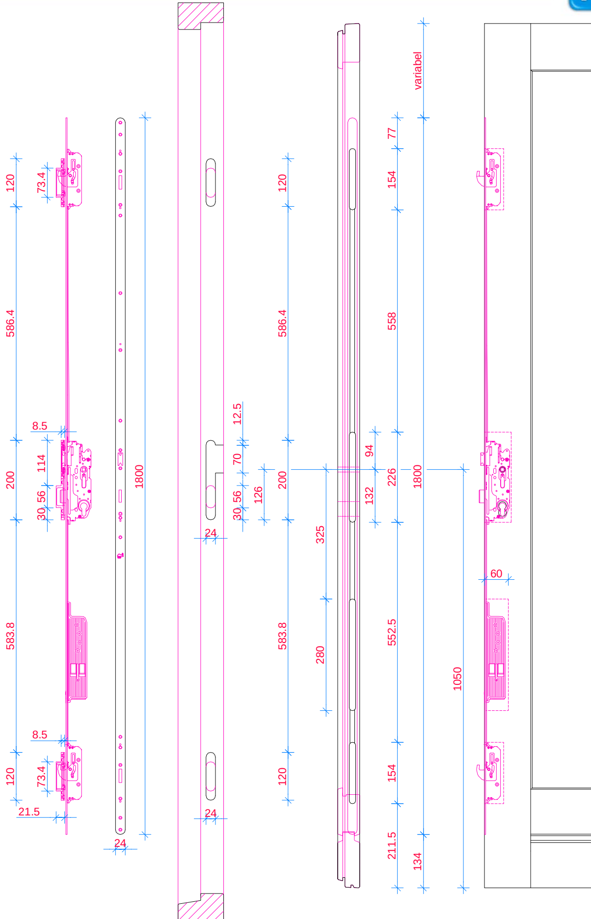
Deur bu/bi draaiend hg 1950-2200 mm - MULTITRONIC 881GL
