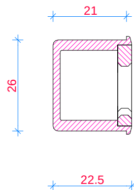
doorsnede B
