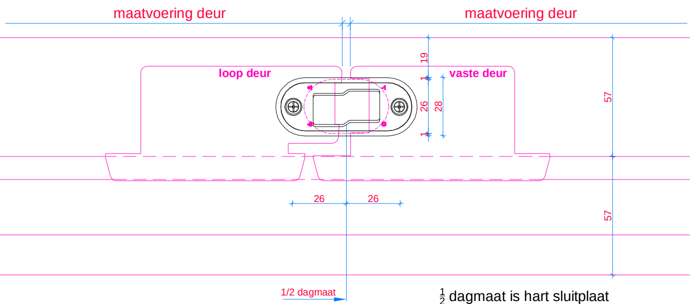
sluitpot recht + sluitplaatje RS56458X
