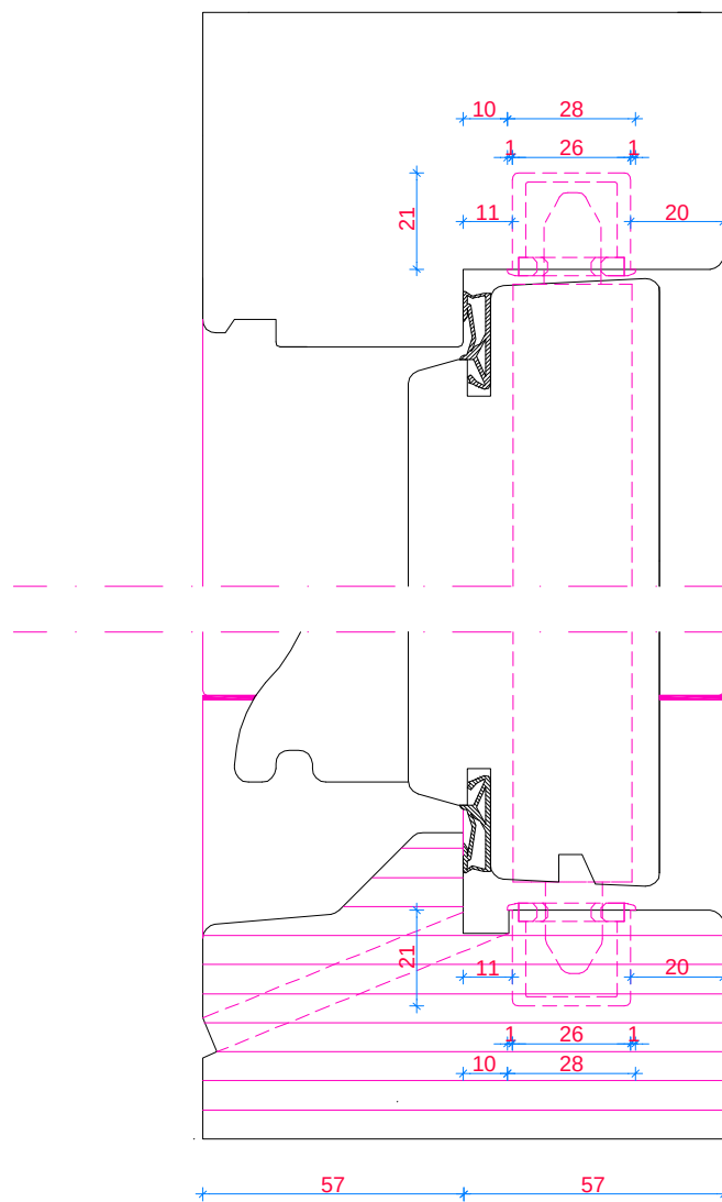
sluitpot recht + sluitplaatje RS56458X
